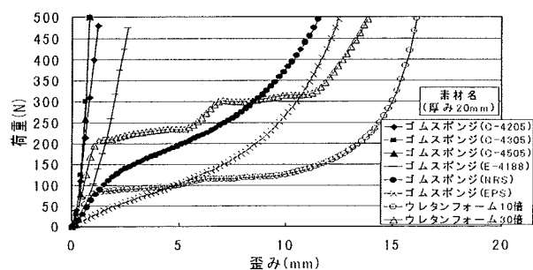
図5 把持素材の荷重-歪み曲線の一例
