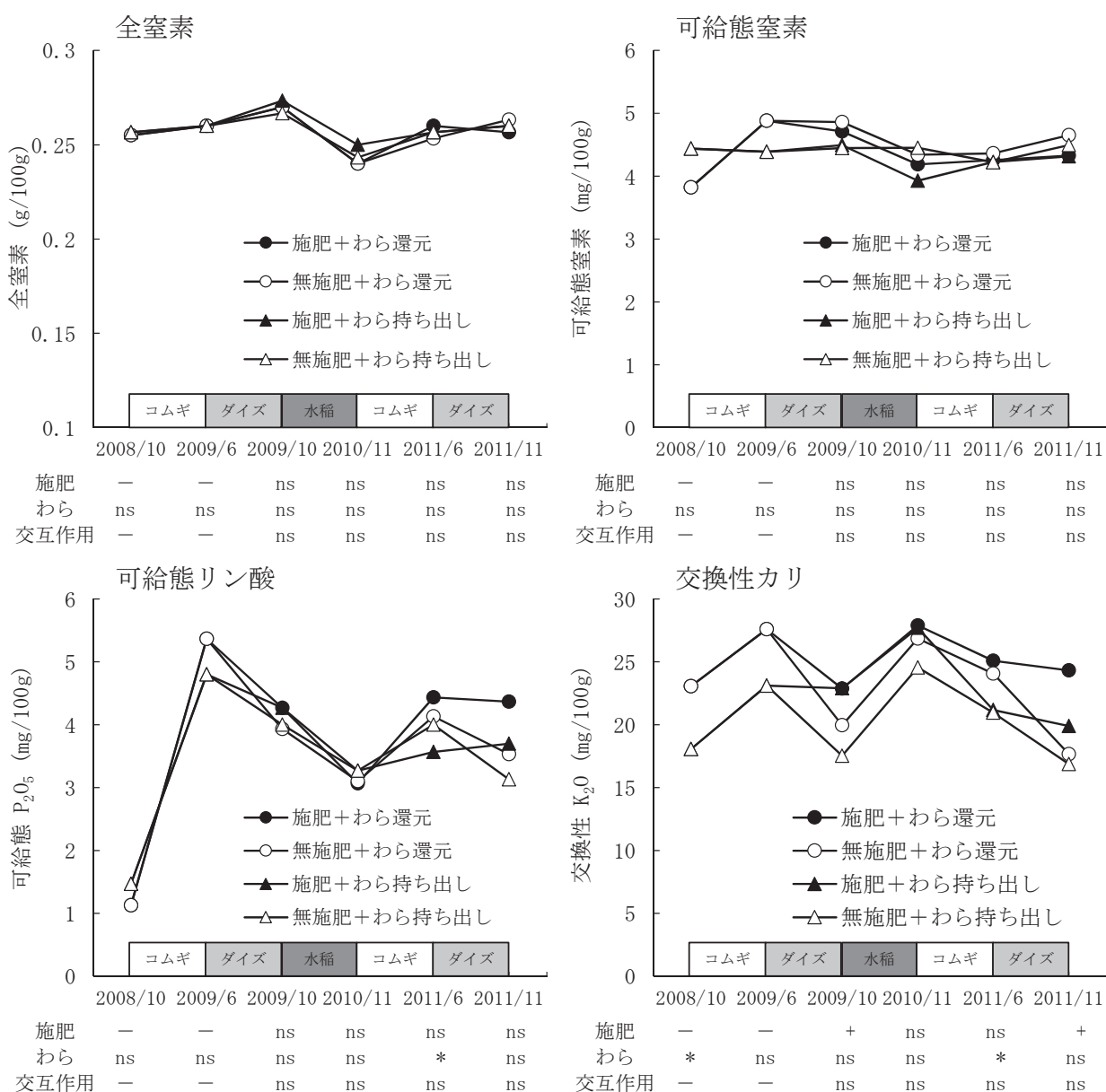
図3 場内試験におけるダイズ栽培時の基肥の有無と稲わら、麦わらの持ち出しの有無が土壌の化学性の推移に及ぼす影響。
