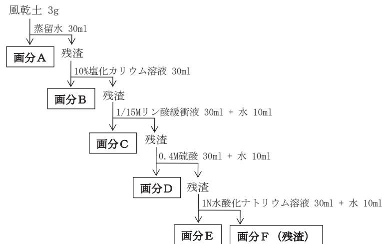
図2 現地試験にてサンプリングした土壌の窒素の逐次抽出手順。
