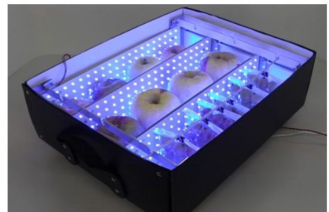
写真1 青白い光を放つ「果実発色促進装置」 （山口県産業技術センター提供）
