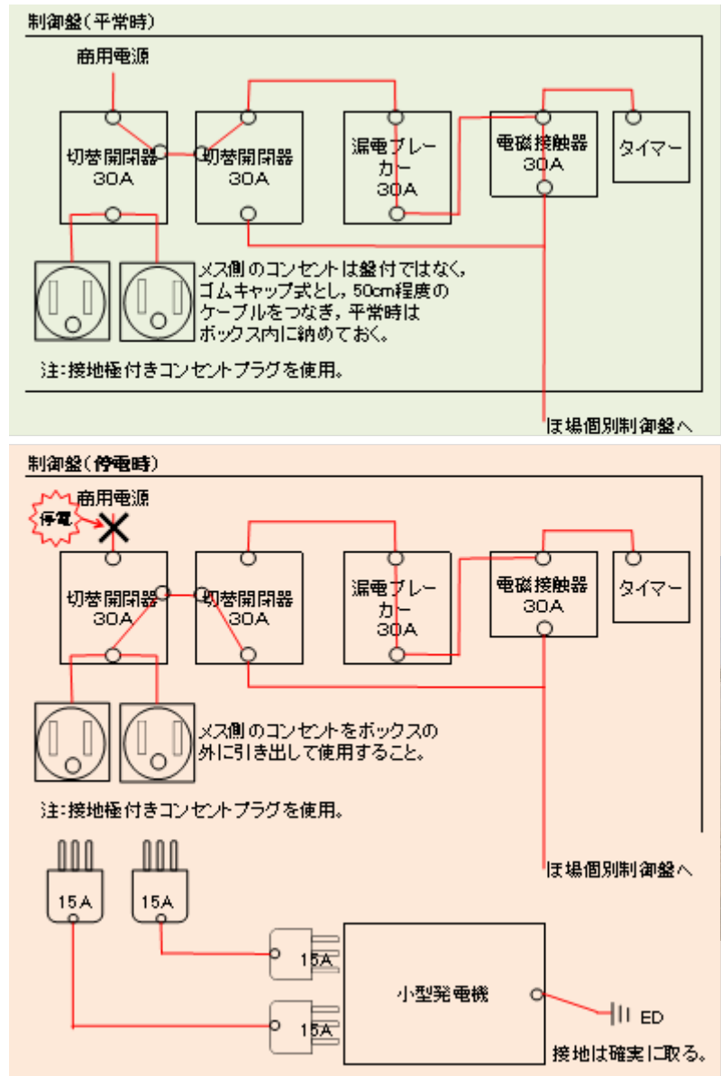
図2 非常用電源ボックスの仕様
