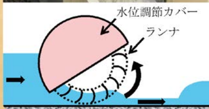
しょうすいりよくはつでん 小水力発電
