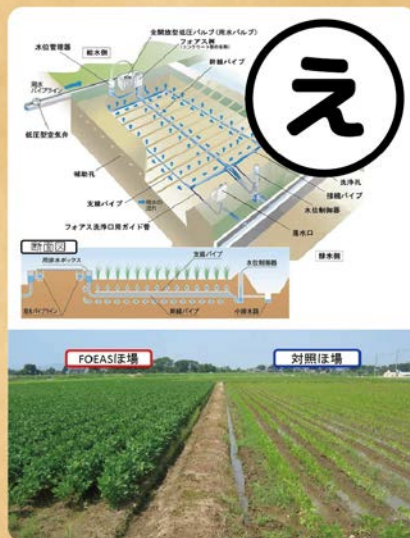
フォアス (地下水水位制御システム) ち か す い い せいぎょ
