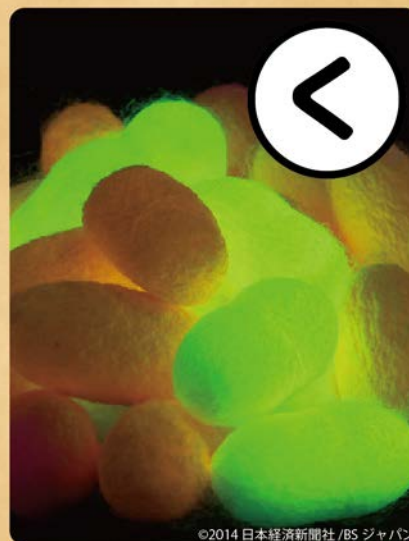
光る繭 (遺伝子組換えカイコ) ひか まゆ いでんしくみか
