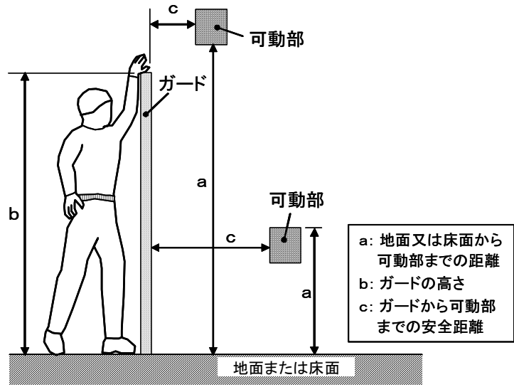
図1 ガードから可動部までの安全距離
