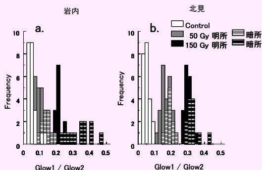
ガンマ線照射した馬鈴薯の貯蔵5ヶ月後のTL比の分布
