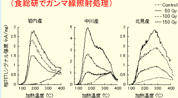
北海道産馬鈴薯に付着した鉱物のTLスペクトル (食総研でガンマ線照射処理)
