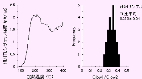
士幌アイントープ照射センターで照射された馬鈴薯から得られた鉱物のTLシグナルおよびTL比の頻度分布
