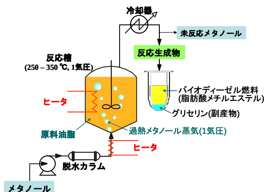
図1 過熱メタノール蒸気法に基づく反応装置の概略
