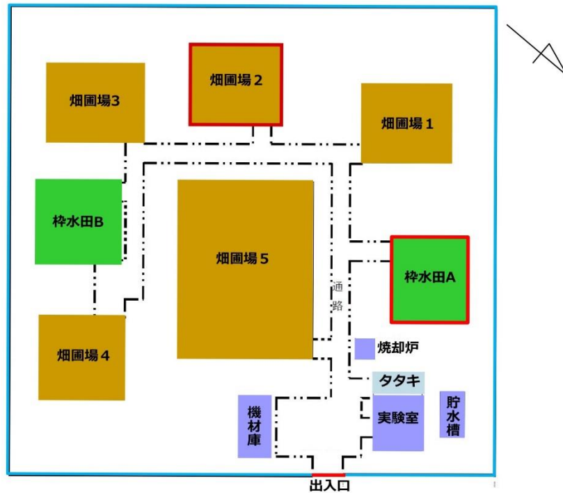
図1 観音台第3事業場組換え植物隔離ほ場場内水田配置図
