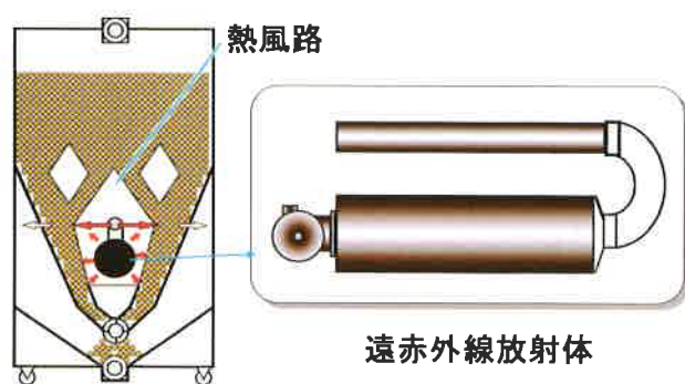
遠赤外線乾燥機の断面図と遠赤外線放射体の配置
