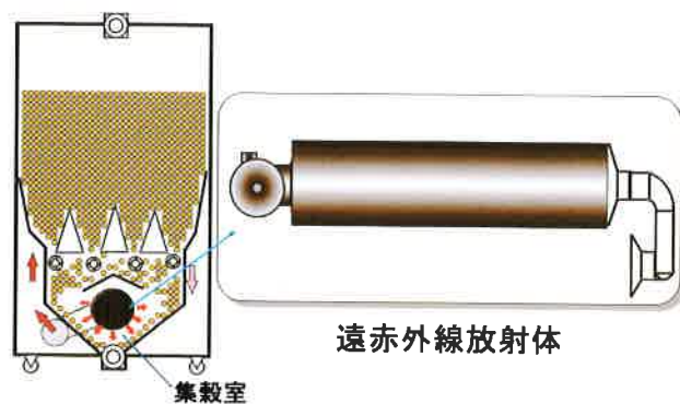
遠赤外線乾燥機の断面図と遠赤外線放射体の配置
