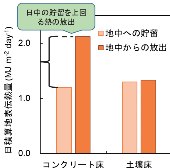
図3 各床材表面での熱の貯留・放出
