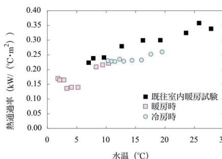
図3 熱通過率
