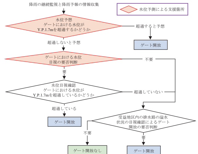
図1 水位調節ゲートの操作フローと水位予測による支援箇所
