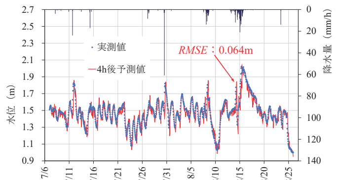
図3 Nearest-Neighbor法による水位予測結果
