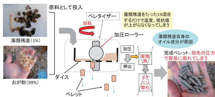
図1 ペレタイザーを適用した藻類残渣ペレット化の試行
