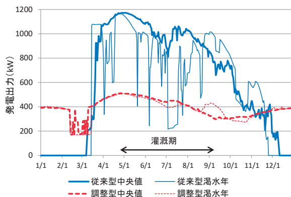
発電出力の経時変化
