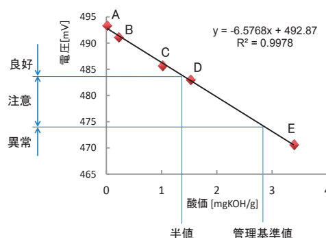
図3 潤滑剤の酸価と電圧の関係 (管理基準値および三段階評価はイメージ)
