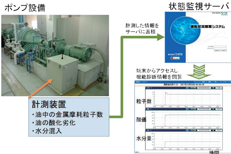
図1 遠隔監視システムの構成
