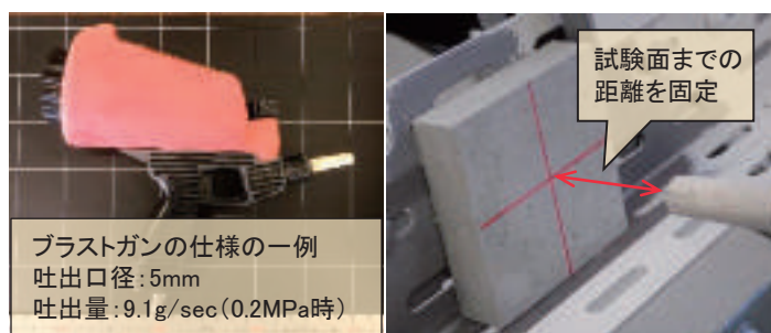
図1 小型サンドブラストと試験状況
