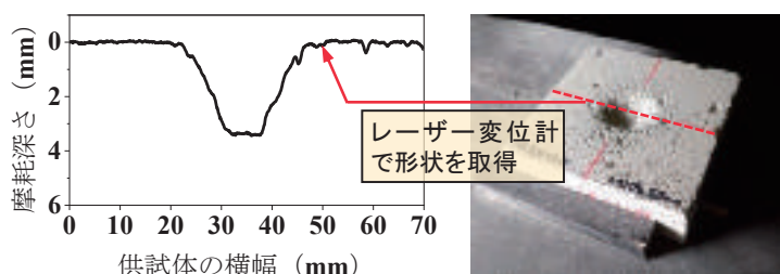
図2 供試体が発生する摩耗形状
