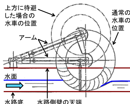
水車の水路上方への待避の設置図
