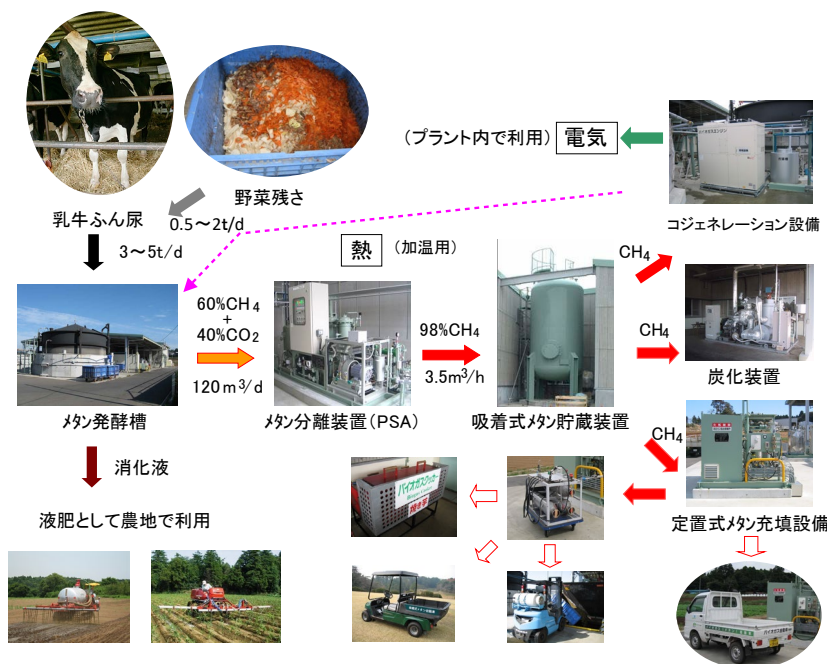
山田バイオマスプラントを核とするメタン発酵システム
