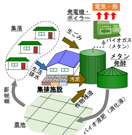
図1 集排汚泥と地域バイオマスのメタン発酵システム
