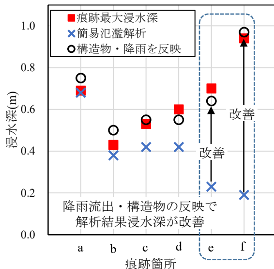
図2 解析結果と痕跡の浸水深比較
