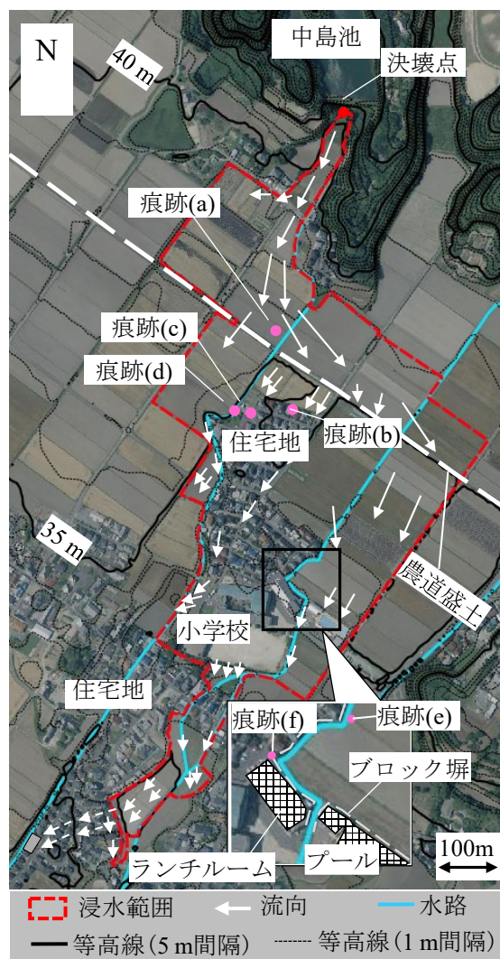
図1 痕跡箇所の位置
