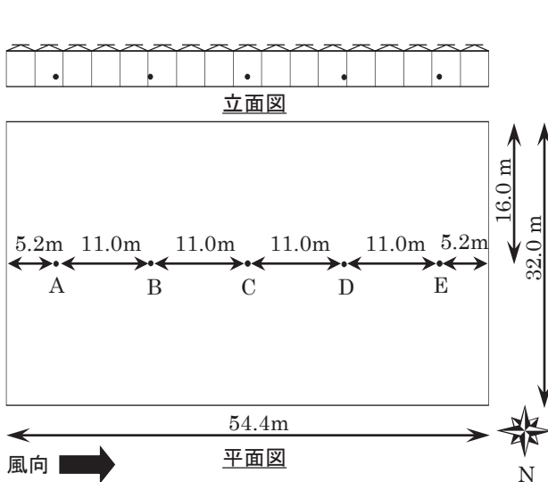
図1 17連棟のフェンロー型温室の平面・立面図および測定点(●)の配置
