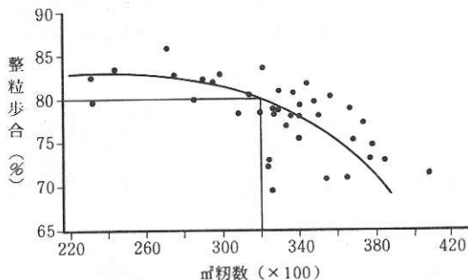
図1 m 2 当たり粗数と整粒歩合
