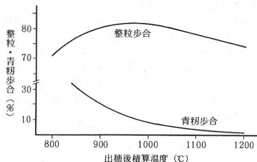
図5 出穂後積算温度と整粒歩合, 青歩合
