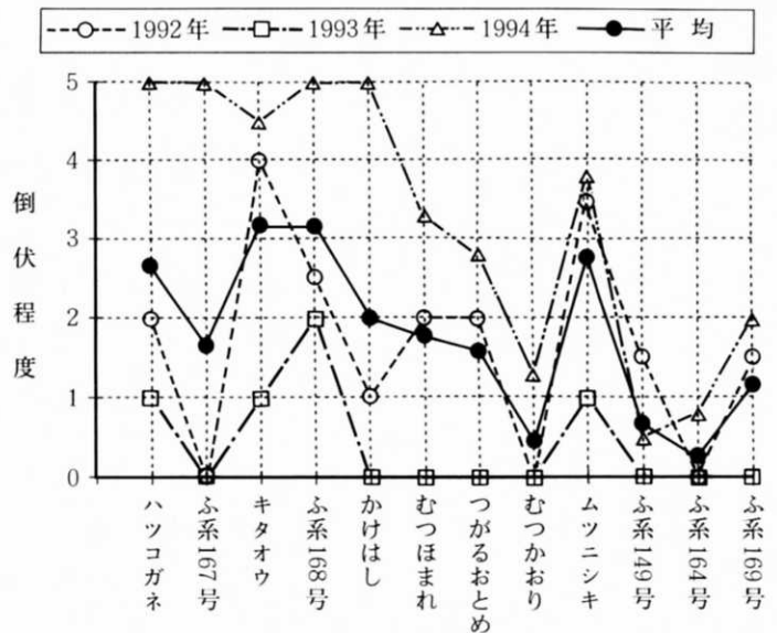
図3 各品種・系統の年次別倒状程度
