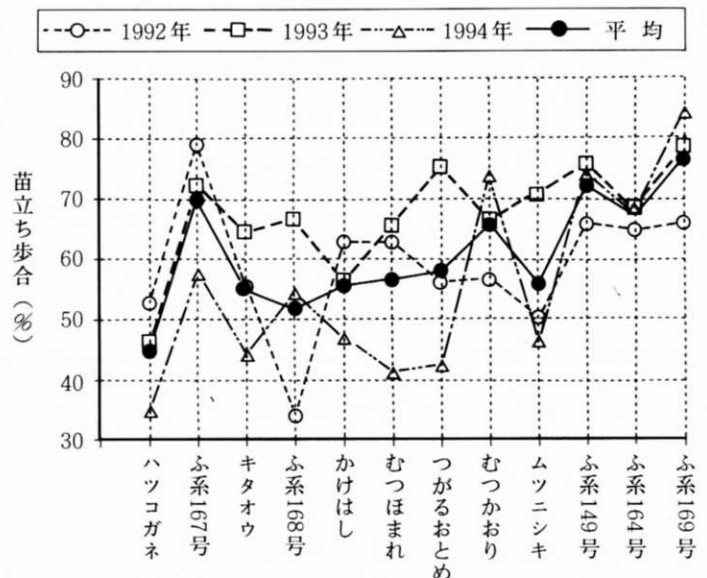
図1 各品種・系統の年次別苗立ち歩合
