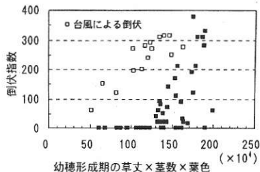
図6 幼穂形成期の生育量と倒伏の関係 (1996～2000年)
