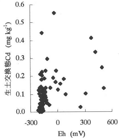
図 1 Eh と交換態 Cd の関係
