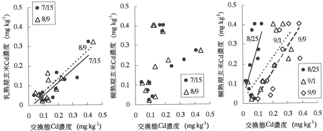
図 5 交換態 Cd と糊熟期の玄米 Cd の関係
