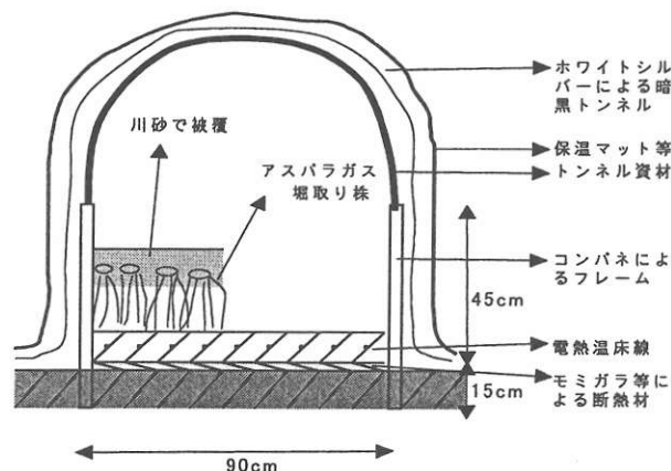
図1 フレームの設置とアスパラガスの伏せ込み略図
