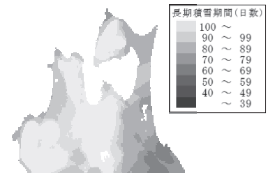
図1 試行1で作成した推定モデル式をもとに作成した長期積雪期間平年値のメッシュ階級図
