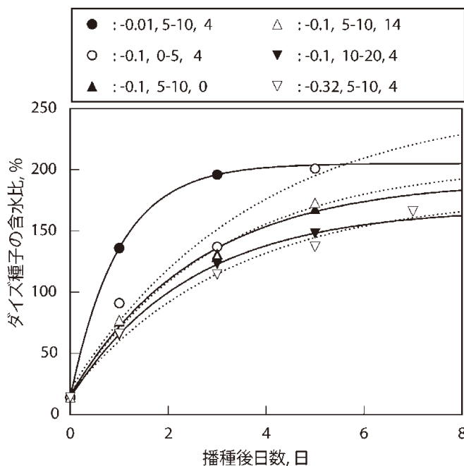
図27 土壤水分ポテンシャル、土塊径、鎮圧強度と播種床におけるダイズ種子の吸水パターンの例(室内実験)
