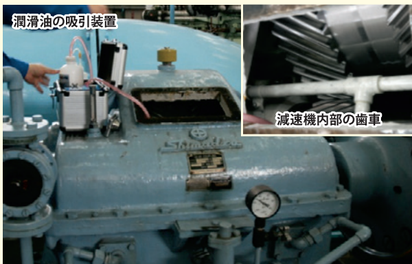
潤滑油に含まれる金属摩耗粒子を分析することで農業水利施設（ポンプ施設）の機能診断を行う技術
