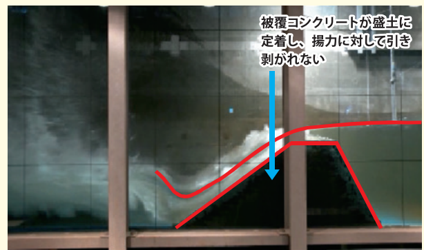
津波に対して粘り強い堤防開発のための模型による水理実験（右側から人工的な津波を作用させた堤防模型の挙動を観察）
