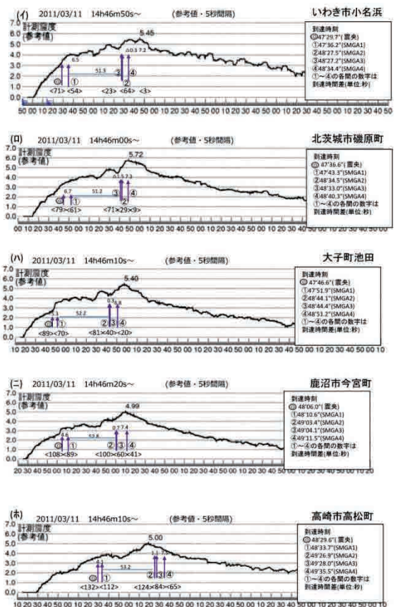
Fig.83 東北地方太平洋沖地震のS2・S3同時ライン(S2=S3+123.3)上観測所の計測震度経過
