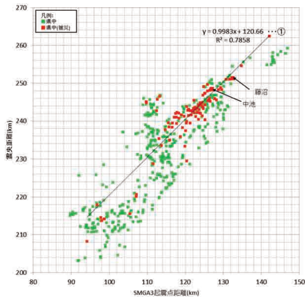
Fig.35 東北地方太平洋沖地震の福島県中被災ため池の震央及びSMGA3距離
