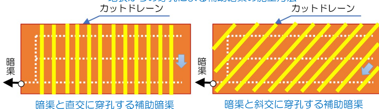
地表からの穿孔による補助暗渠の施工方法
