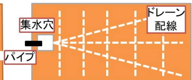
集水穴からの施工時の配線の例
