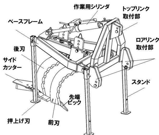
カットドレーンの構造
