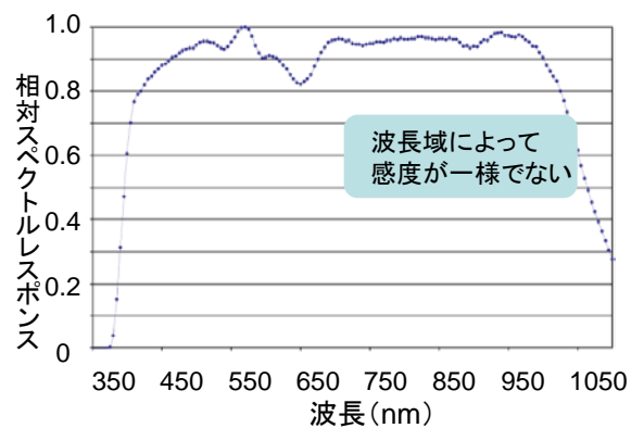
放射照度計センサーの分光反応(あるセンサーの例)
