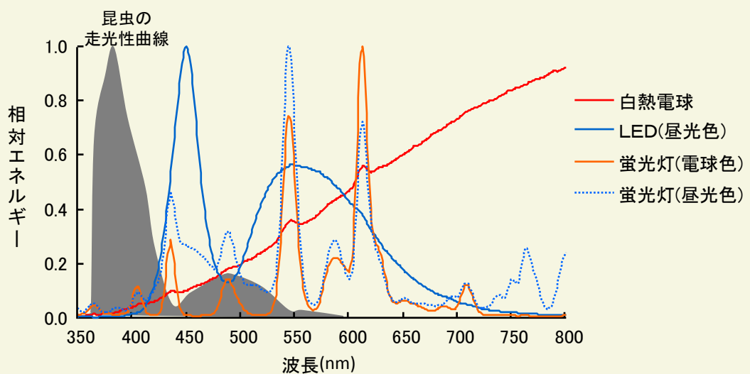
図 各電照用光源の波長特性と昆虫の走光性
