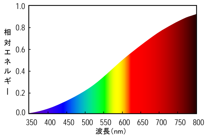
図 白熱電球の波長スペクトル
