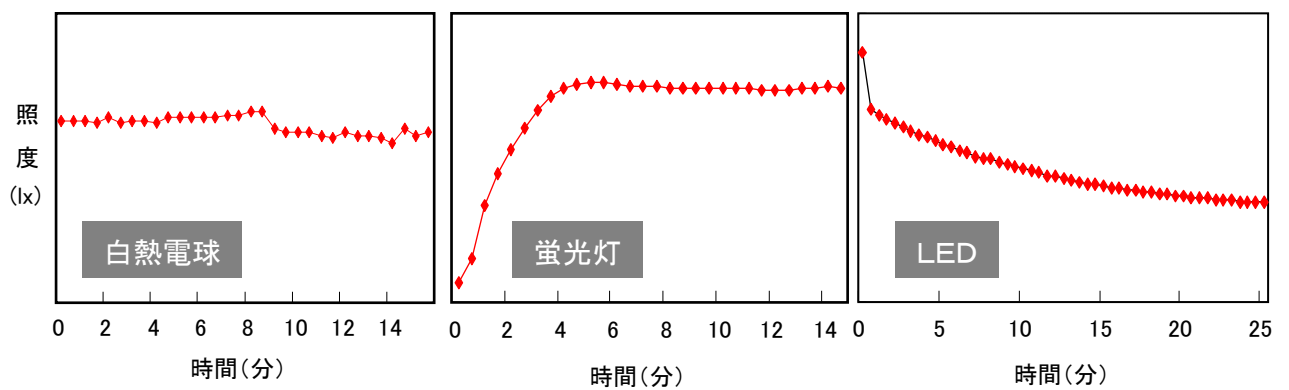
図 光源の種類別、点灯後の照度推移
