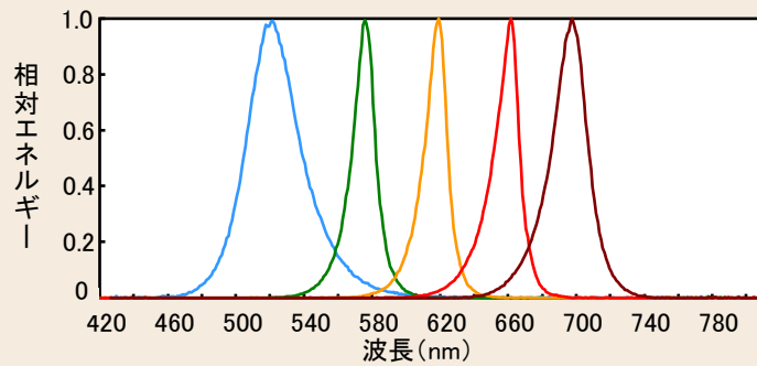
図1 様々な色のLEDの分光分布の例
