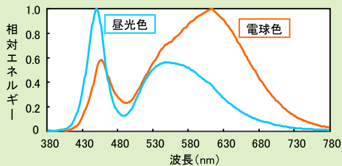
図2 昼光色LED(蛍光体方式)と電球色LED(蛍光体方式)の分光分布の例
