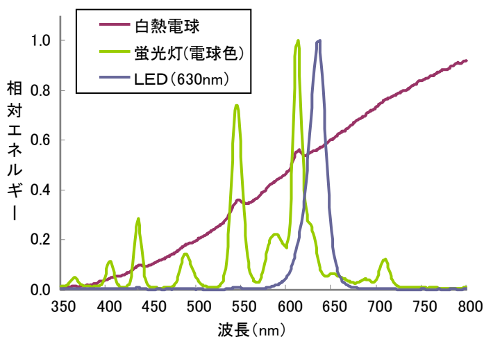
図 分光放射照度計を用いて測定された分光分布図
