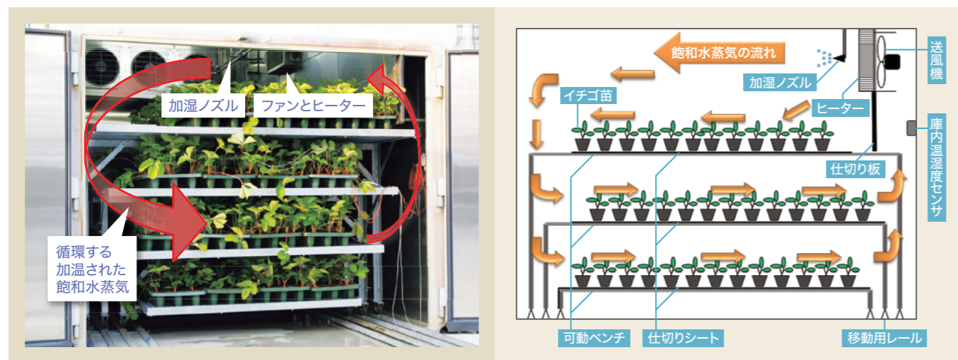
図2 夜冷蔵庫一体型 大型蒸熱処理防除装置 夜冷蔵庫の写真の奥に写っている3個のファンは冷蔵装置のもの。その右に蒸熱処理用の加湿ノズルの配管とヒーターの四角い囲いの一部が見える。蒸熱の気流は模式図のように流れる。
