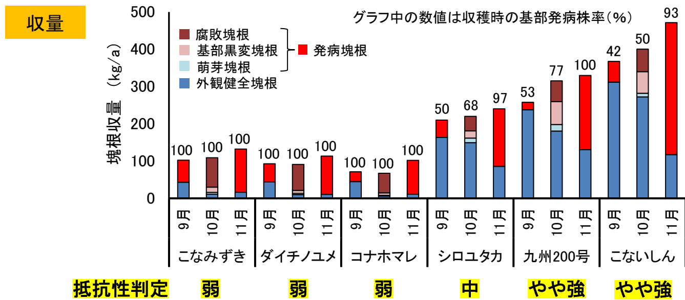
図14でん粉原料用品種の基部発病株率の推移(上)と発病程度別塊根収量(下)(農研機構九冲研) 基腐病甚発生圃場にベンレート処理した苗を植え付け(2021年5月8日、30株3反復)、株基部の発病を経時的に調査し、10月(栽培期間159日)には塊根の発病程度および収量を調査した。また、同様に苗を植え付け(10株3反復)、9月(栽培期間119日)および11月(栽培期間183日)に株基部および塊根の発病の有無と収量を調査した。
