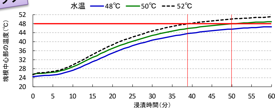
図32 水温の異なる温湯浸漬による塊根中心部の温度推移
