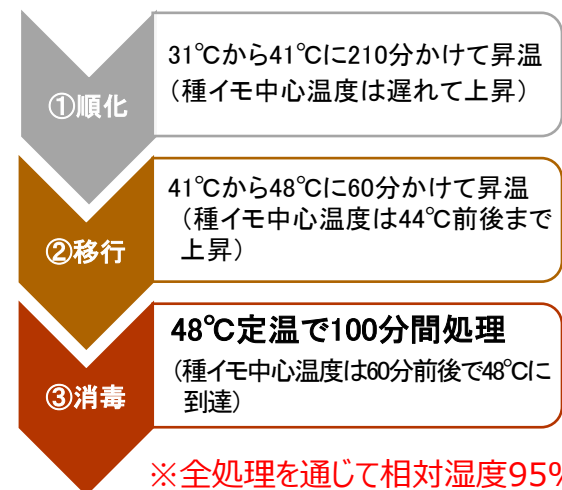
図34 生産現場に実装された蒸熱処理プログラム例
