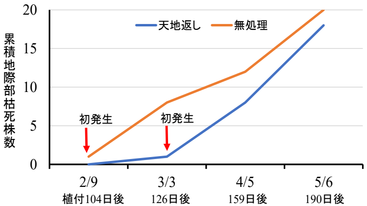
図64 天地返し(70cm)による基腐病防除効果 (沖縄農セ)
