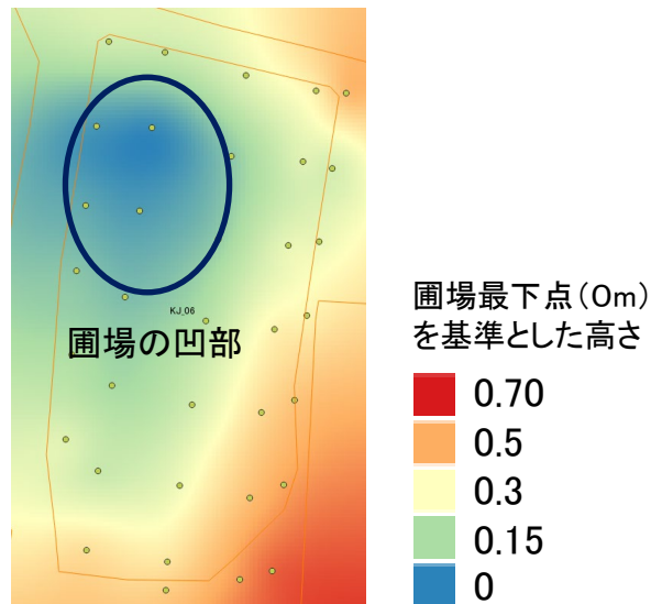
圃場の表面標高(測量)図
