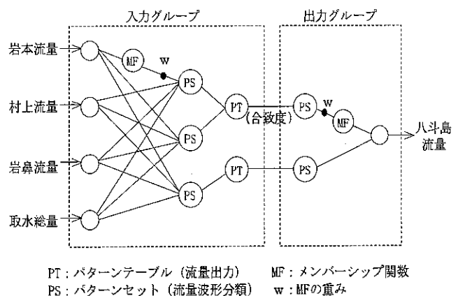
Fig. 5 ファジィ化ニューラルネットによる流量予測と入出力例 (例えば, 八斗島流量予測)
