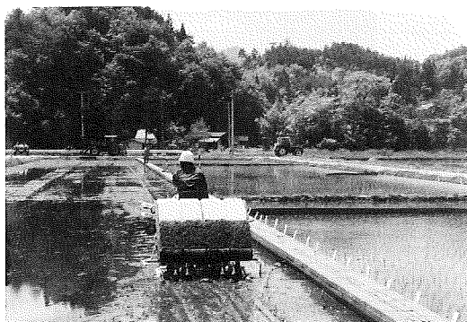
図1 超高速植付試験
