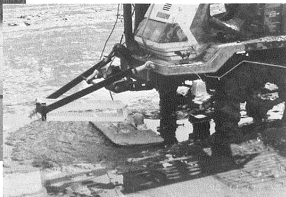
図2 前センサ取付部
