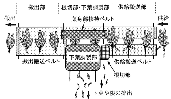
図1 軟弱野菜調製機の概要図
