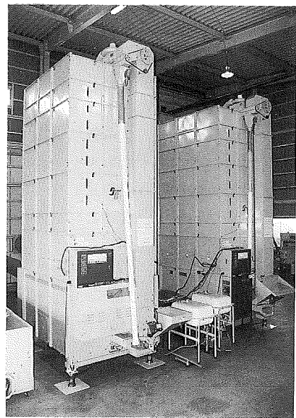
図2 穀物遠赤外線乾燥機の例（左側）
