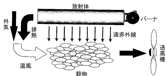
図3 穀物遠赤外線乾燥機での熱エネルギーの流れ
