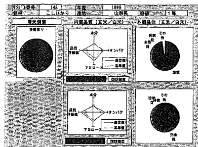
図4 米品質測定評価装置の表示例
