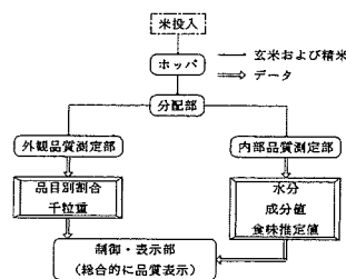
図2 米品質測定評価装置II型
