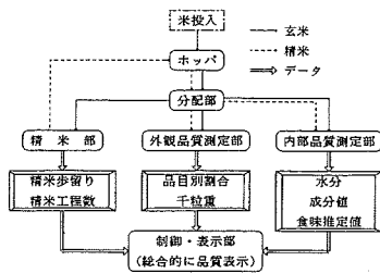
図1 米品質測定評価装置I型
