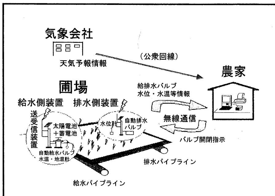
図 水田の自動水管理システム
