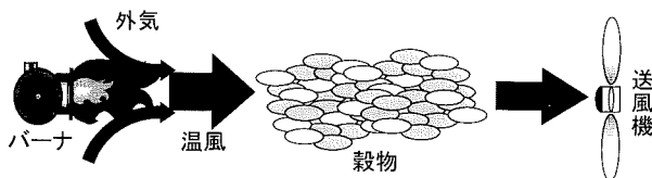
図1 循環式熱風乾燥機での熱エネルギーの流れ
