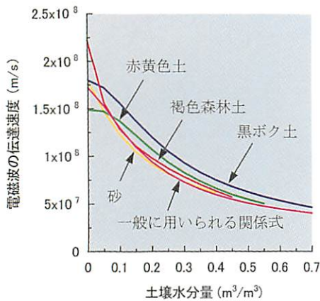
図1. 九州沖縄地域の土壌の電磁波伝達速度と土壌水分量の関係
