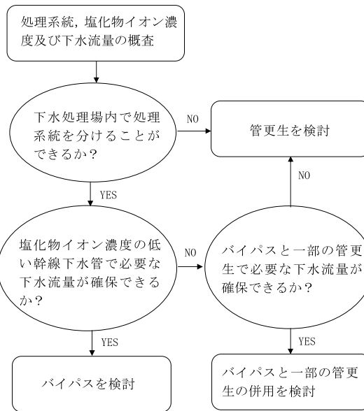
Fig.28 塩分低下対策の指針
