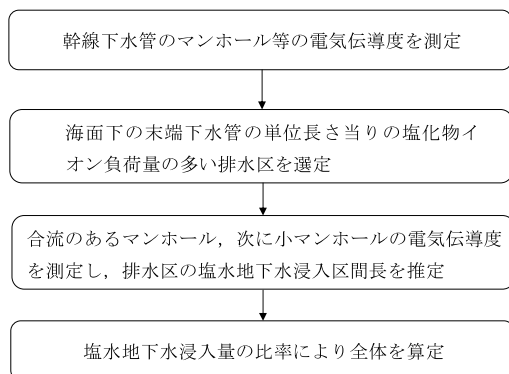
Fig.29 塩水地下水浸潤区間長の推定手法
