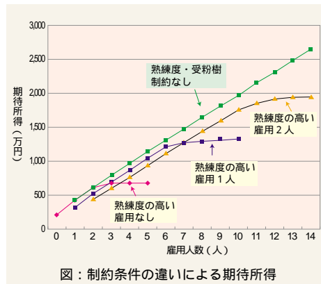
図：制約条件の違いによる期待所得
