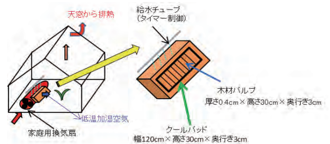
第1図 簡易設置型パッドアンドファン冷房システムのしくみ
