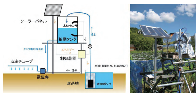
図1 日射制御型拍動自動灌水装置と設置例
