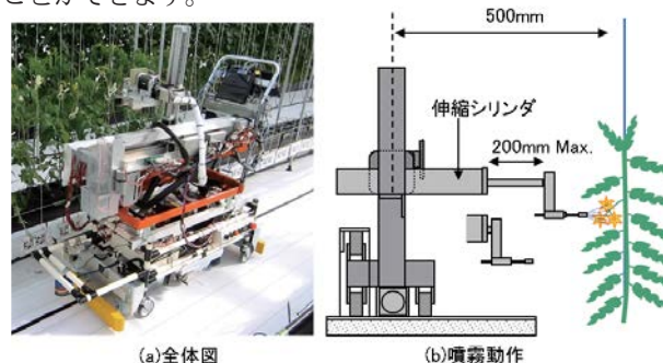
図2 ロボットの外観とホルモン剤噴霧動作
