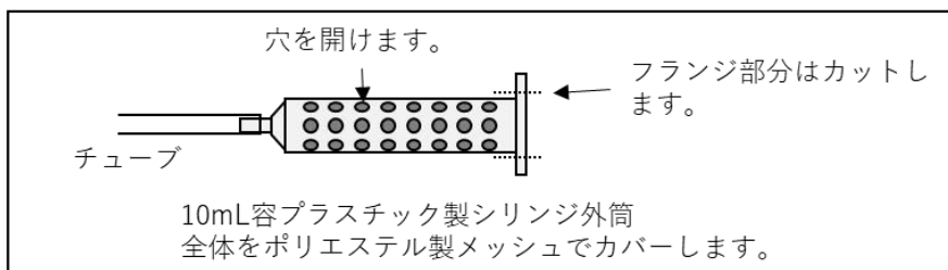
図 2-7 GEA 社 MIOne（農研機構）での設置例
