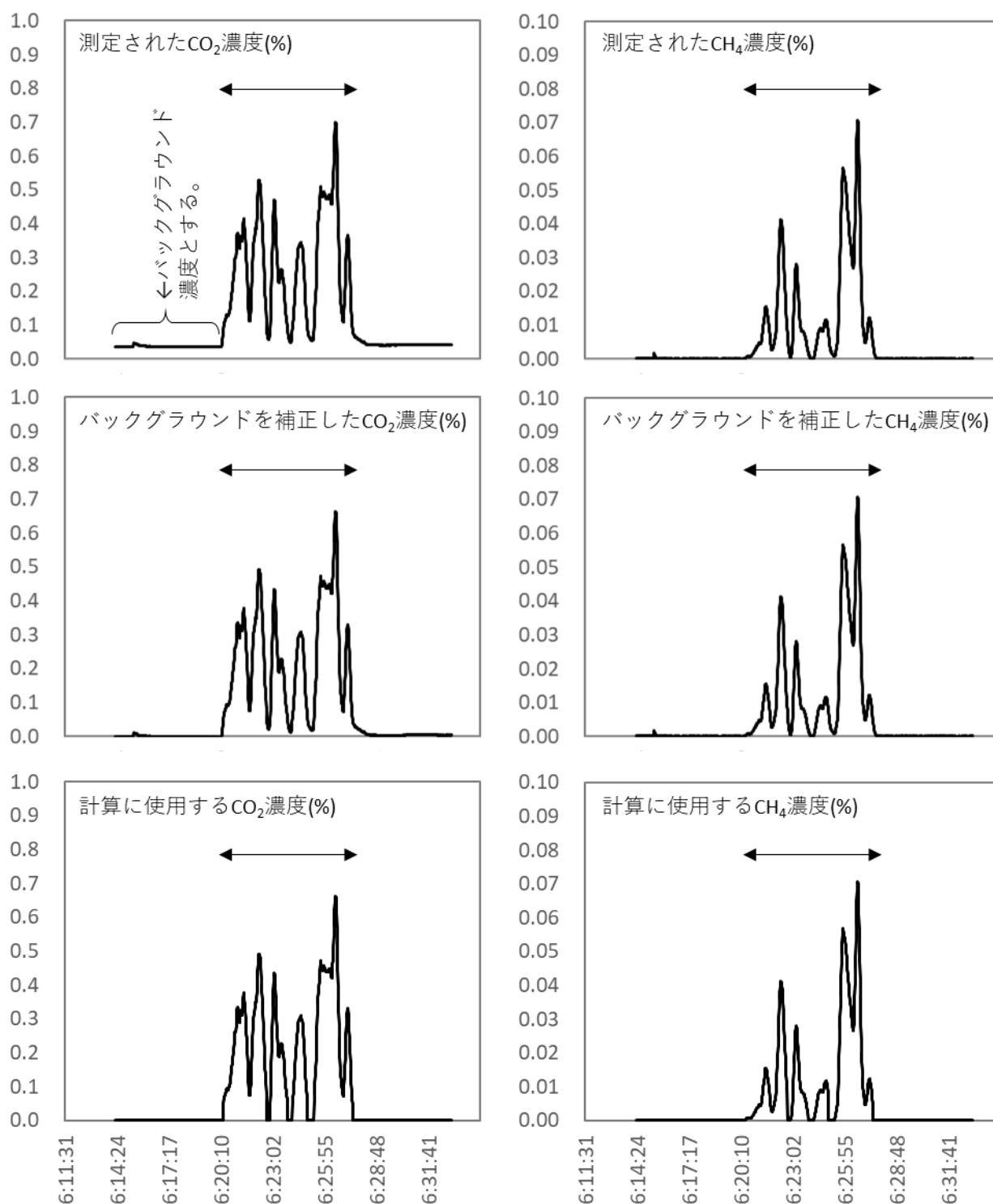
図 2-10 \text{CH}_4/\text{CO}_2 比算出に使用する \text{CO}_2 濃度（左列）と \text{CH}_4 濃度（右列）の例 ガス分析計出力（上段）、バックグラウンド濃度を差し引いた後のガス濃度（中段）、および計算に使用するガス濃度（下段）。矢印の期間は乳牛一頭が搾乳されていた期間を示す。
