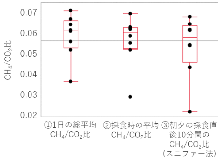
図 3-4 算定方式の違いによる \text{CH}_4/\text{CO}_2 比の比較 図中の横線は全体の平均値を示す。
