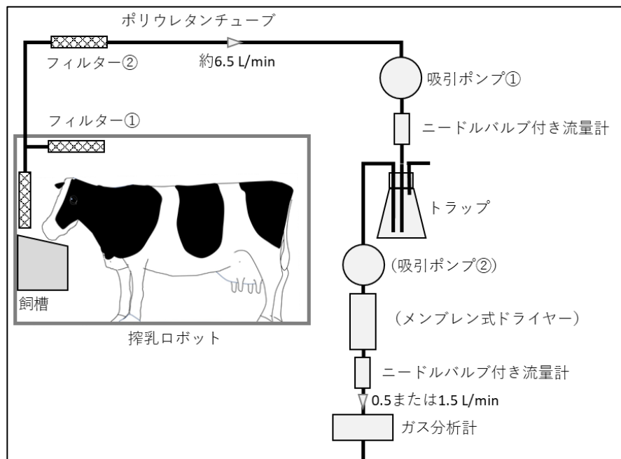
図 2-1 測定システム概要（トラップ有り）
