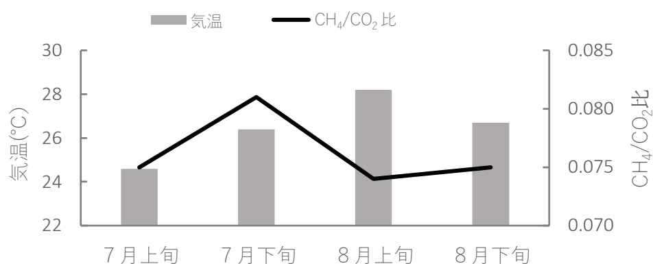
図 2-12 夏季の進行に伴う気温と \text{CH}_4/\text{CO}_2 比の変化
