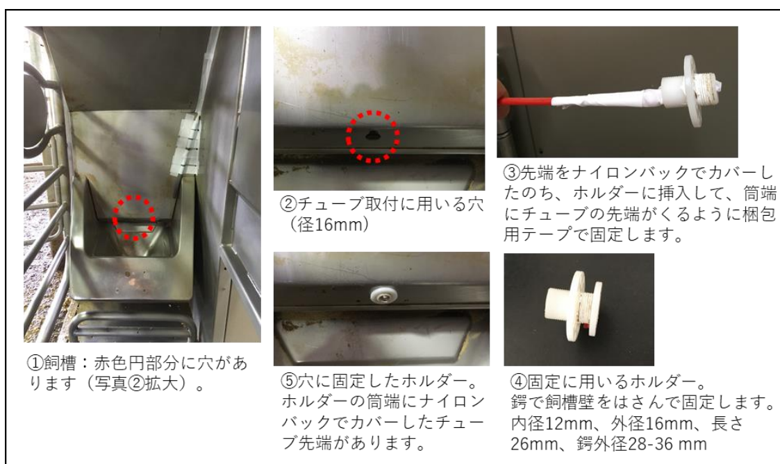
図 2-6-2 Lely 社 Astronaut A3 Plus（広島大学）での設置例 飼槽の飼料投下口上縁（黄色円部分）にある穴を利用してチューブを固定する方法。
