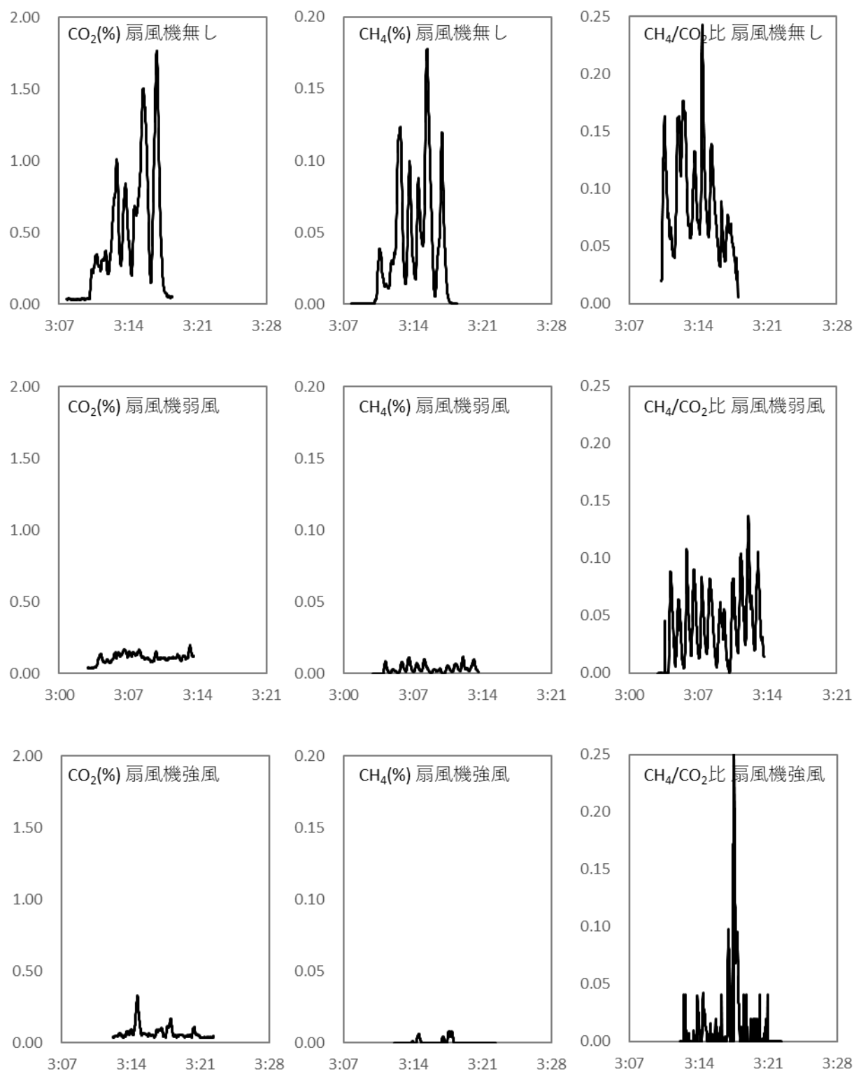
図 2-9 搾乳ロボットに小型扇風機で送風したときの \text{CO}_2 濃度 (左)、 \text{CH}_4 濃度(中)、および補正後 \text{CH}_4/\text{CO}_2 比 (右)
