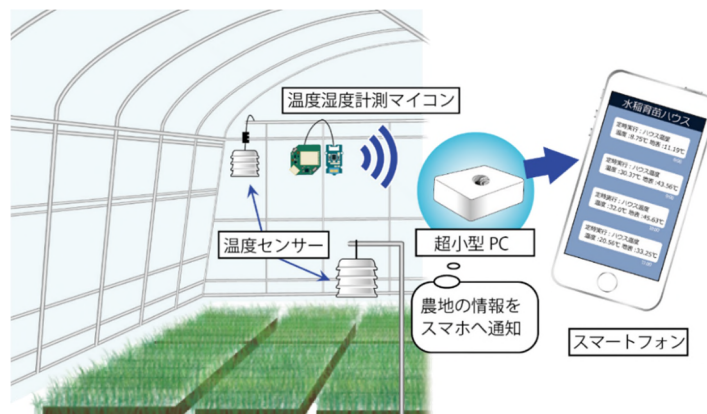
図1 通い農業支援システムのイメージ
