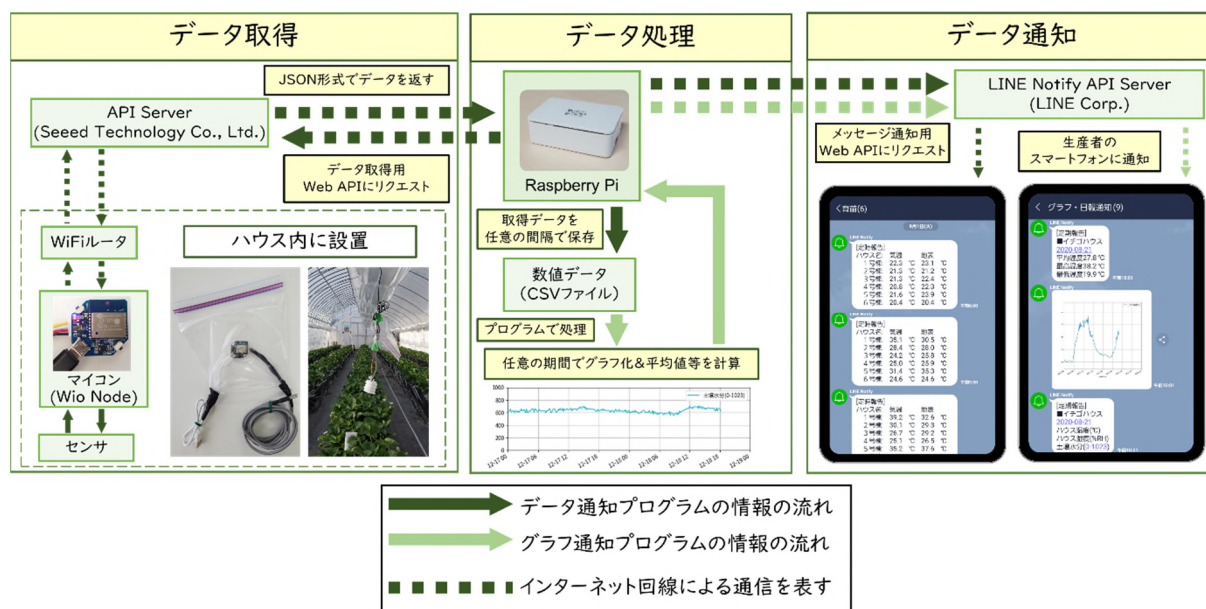
図8 「通い農業支援システム」の仕組み
