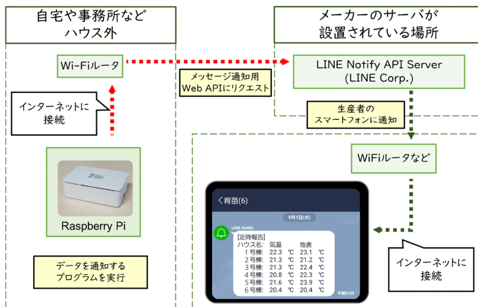
図6 メッセージ通知の仕組み
