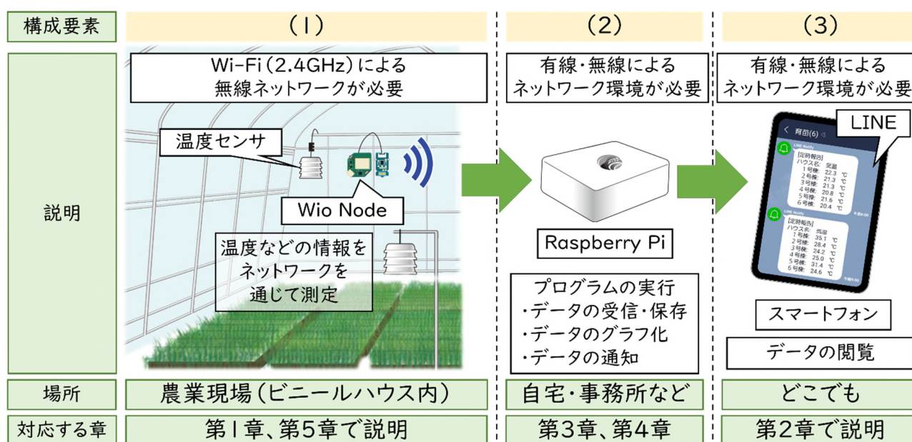
図2 通い農業支援システムの構成要素とその役割
