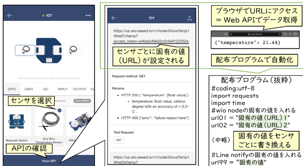
図5 データ取得用 Web API のアクセストークンの設定方法と自動化方法
