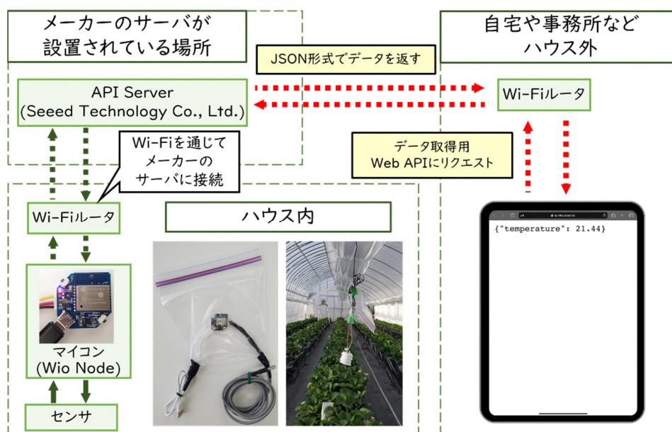
図4 Web API を利用したデータ取得の仕組み
