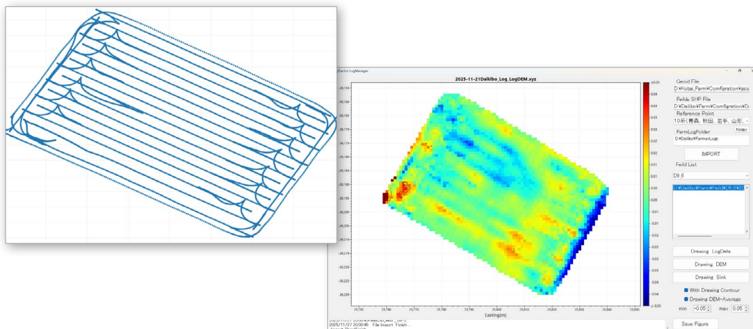
作業軌跡から変換した圃場内凹凸分布例 (左が作業軌跡、右の凹凸マップでは赤が高く、青が低い)
