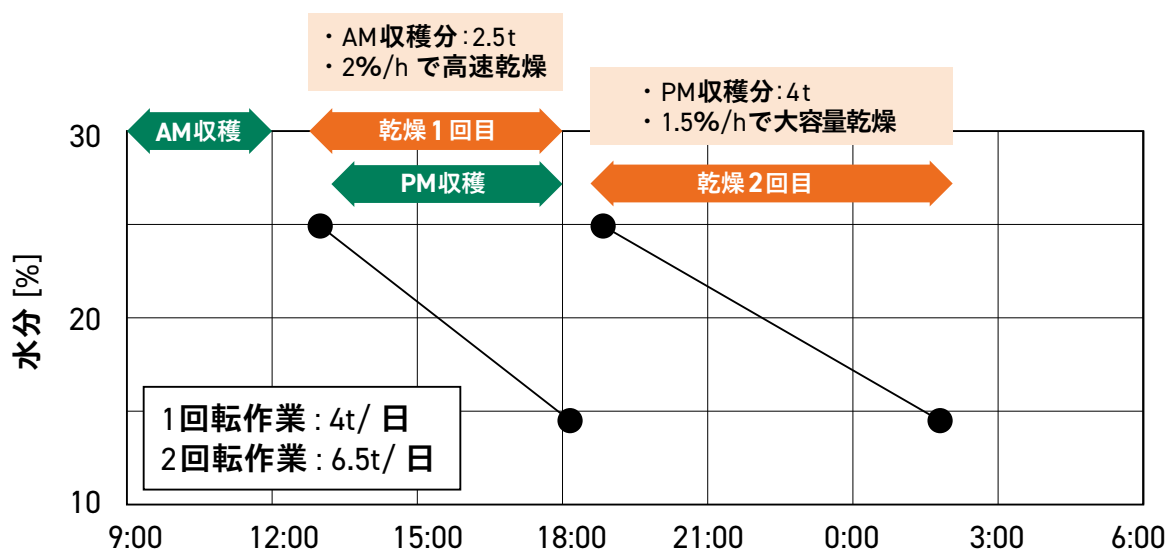
図3 容量4t 乾燥機の2回転運転スケジュール例
