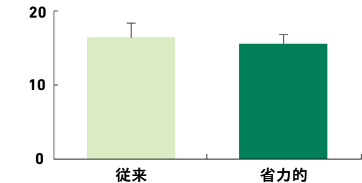
図3 従来および省力的播種床造成技術における畝立て播種後の畝の高さ(cm) 福島県南相馬市の生産者圃場におけるデータ(令和5年) 図中のバーは標準偏差(n=4)
