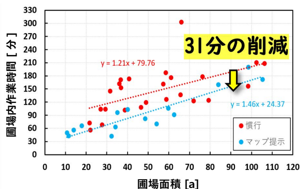
圃場凹凸マップ提示による作業時間削減効果
