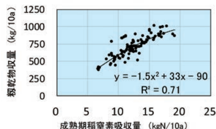
稲窒素吸収量と籾収量の関係 (栽培品種「まなむすめ」)
