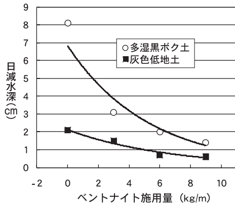
ベントナイト量と日減水深の関係
